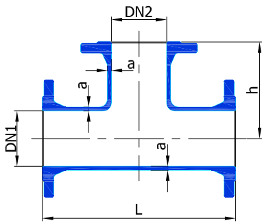
FLANGE - FLANGE TEE
